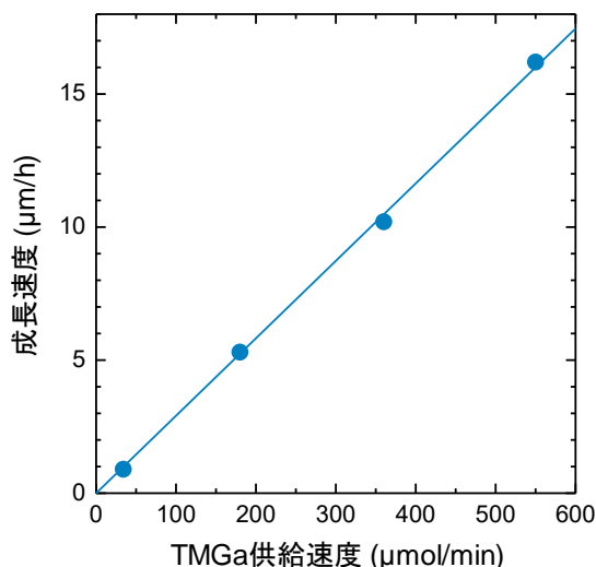
図3 : \beta -Ga 2 O 3 のホモエピタキシャル成長速度の TMGa 供給速度依存性。TMGa 供給速度の増加に対して成長速度は線形に増加する。TMGa 供給速度 550 μmol/min の時に、成長速度は 16.2 ミクロン毎時の高速度となることが分かる。
