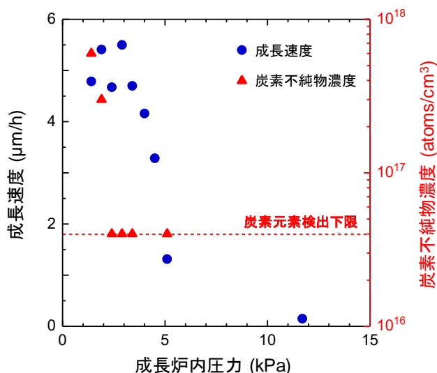
図2 : \beta -Ga 2 O 3 の成長速度および成長膜中の炭素不純物濃度の成長炉内圧力依存性。1000℃にて、TMGa 供給速度 180 μmol/min、O/Ga 供給比 970 で成長。炉内圧力 2.4~3.4 kPa において約 5 ミクロン毎時の成長速度かつ低炭素不純物濃度が両立されることが分かる。
